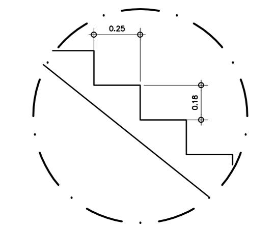
DETALHE ESCADA À LEGALIZAR SEM ESCALA
